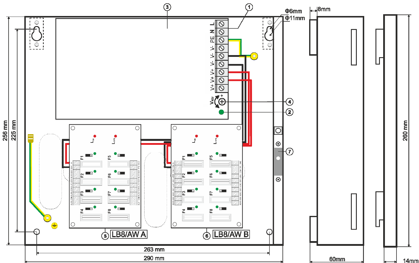
Bild. 3. Netzteil-Ansich.
