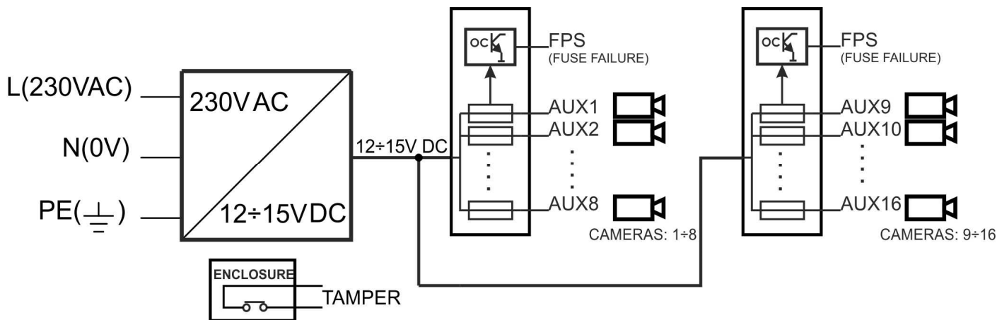
Bild.1. Schaltplan Netzteil.
